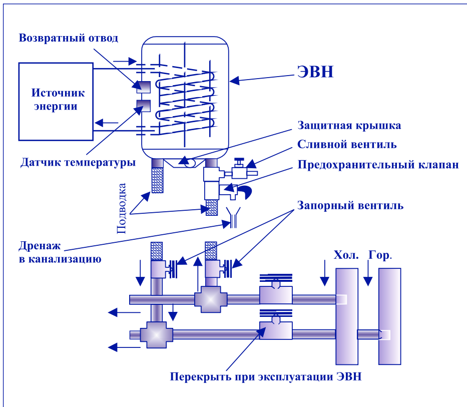
Рис. 1. Схема подключения ЭВН к водопроводу
